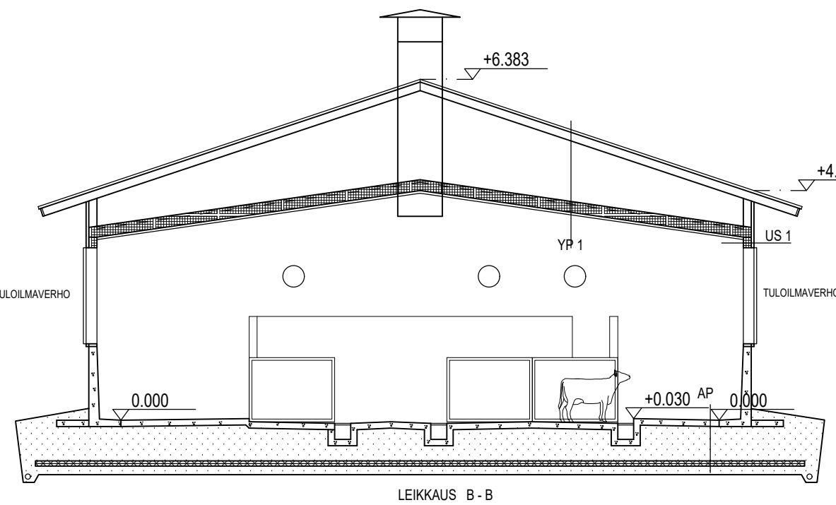
LEIKKAUS B - B
