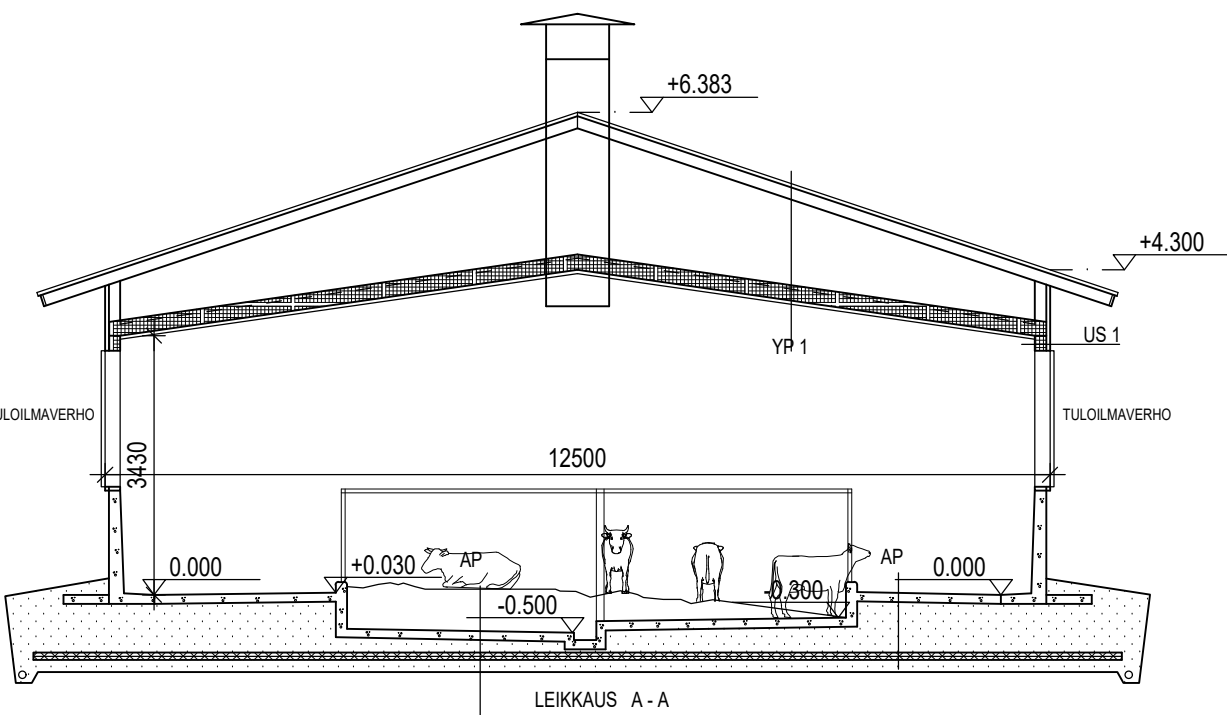
LEIKKAUS A - A
