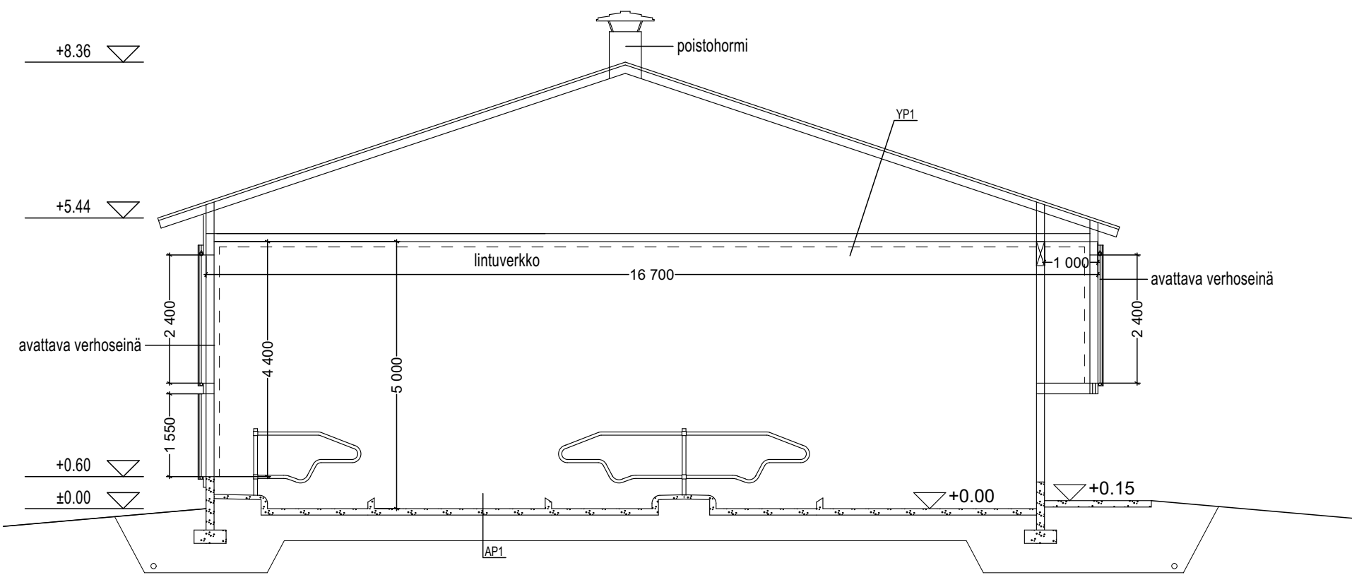
LEIKKAUS A-A
