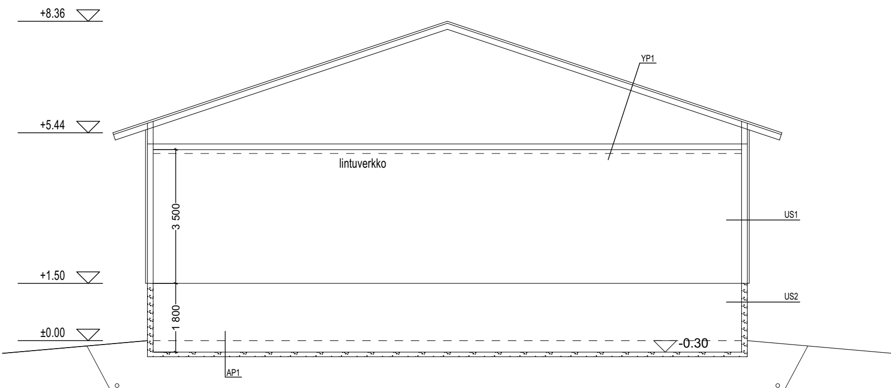
LEIKKAUS B-B
